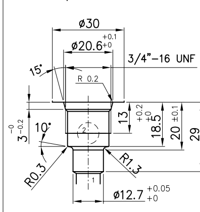
dettaglio sede valvola VEI détail implantation valve VEI
